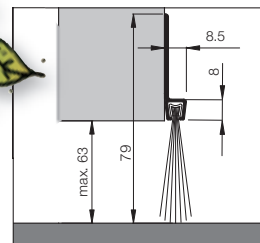
Dollex4 - 80 Art.-Nr. 031-80-sw Bürstenhöhe 39 mm Gesamthöhe 79 mm
