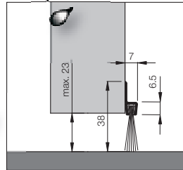
Dollex4 - 40 Art.-Nr. 031-40-sw Bürstenhöhe 20 mm Gesamthöhe 38 mm
