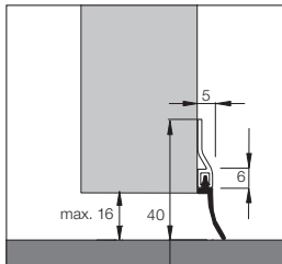
Dollex5 - 16 Art.-Nr. 031-14-sw Lippenhöhe 16 mm Gesamthöhe 40 mm
