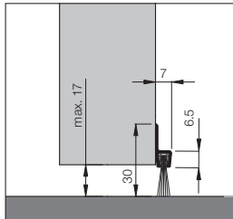
Dollex4 - 32 Art.-Nr. 031-32-sw Bürstenhöhe 12 mm Gesamthöhe 30 mm
