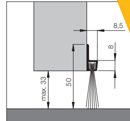
Dollex4 - 50 Art.-Nr. 031-50-sw Bürstenhöhe 30 mm Gesamthöhe 50 mm
