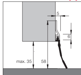
Dollex5 - 35 Art.-Nr. 031-13-sw Lippenhöhe 35 mm Gesamthöhe 58 mm
