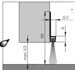
Dollex4 - 70 Art.-Nr. 031-70-sw Bürstenhöhe 29 mm Gesamthöhe 69 mm
