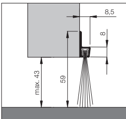
Dollex4 - 60 Art.-Nr. 031-60-sw Bürstenhöhe 39 mm Gesamthöhe 59 mm
